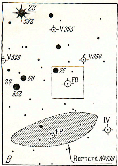
FO Aql
