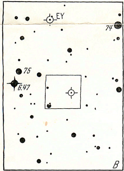
KX Aql
