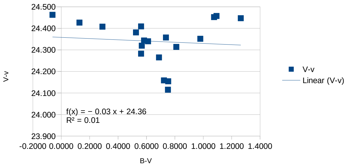
V mag transform V-v vs B-V
