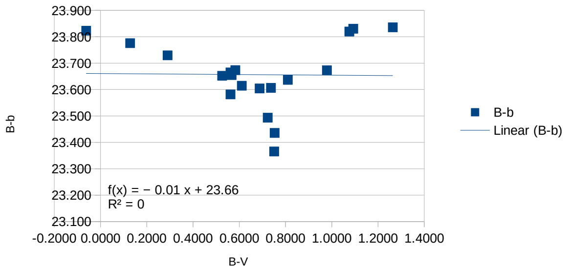
B mag transform
